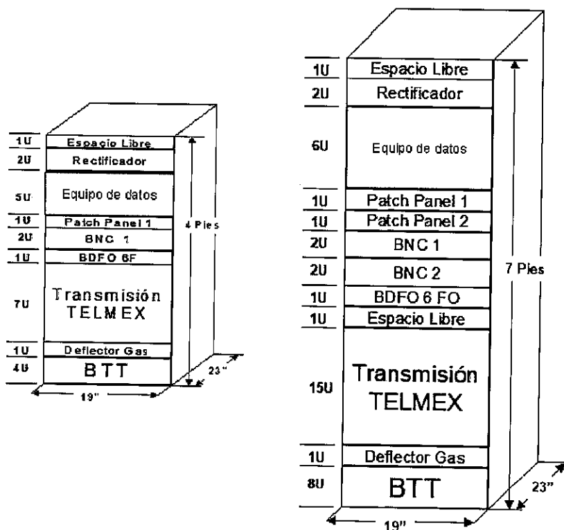
Distribución del gabinete universal Telmex/Telnor
