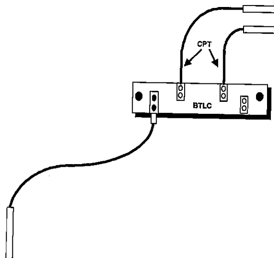
Conexión de Conductores en Cascada.
