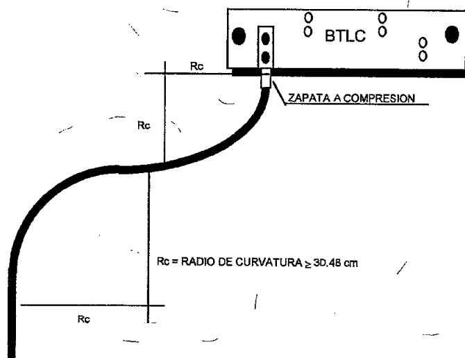
Radios de Curvatura Permisibles
