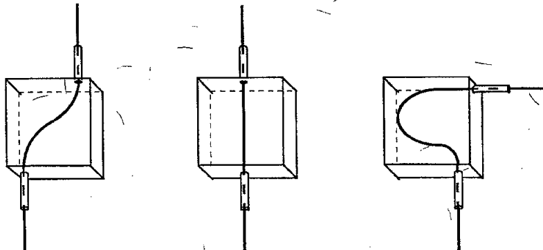
Colocación incorrecta de registros para Fibra óptica.
