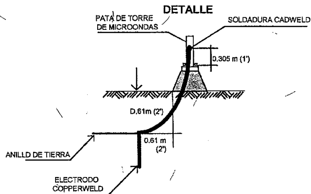
Torres Instaladas a Nivel de Piso.
