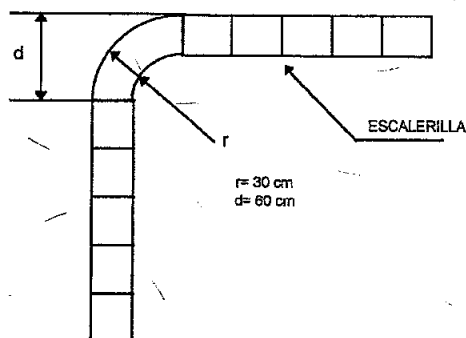
Canalización de Fibra óptica por Charóla o Escalerilla de Cables.
