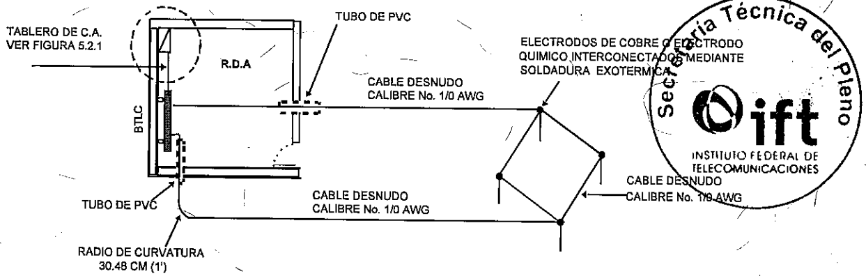
Puesta a Tierra del sitio cliente.
